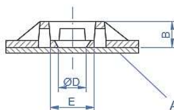
Sección A-A
